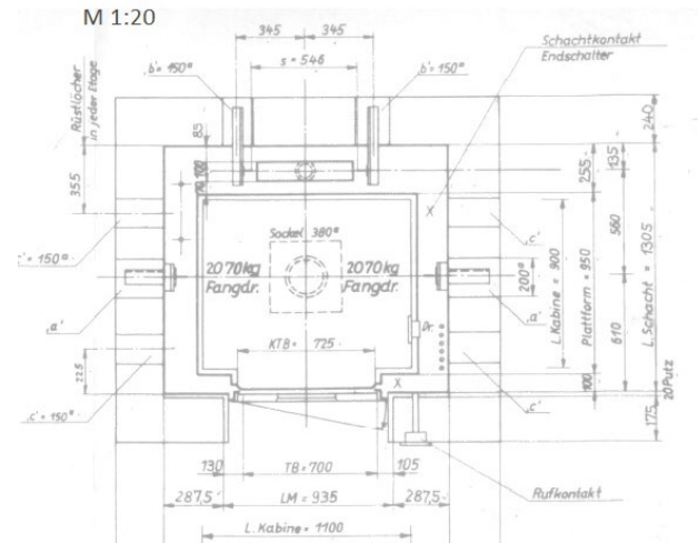
Schacht- Grundriß
