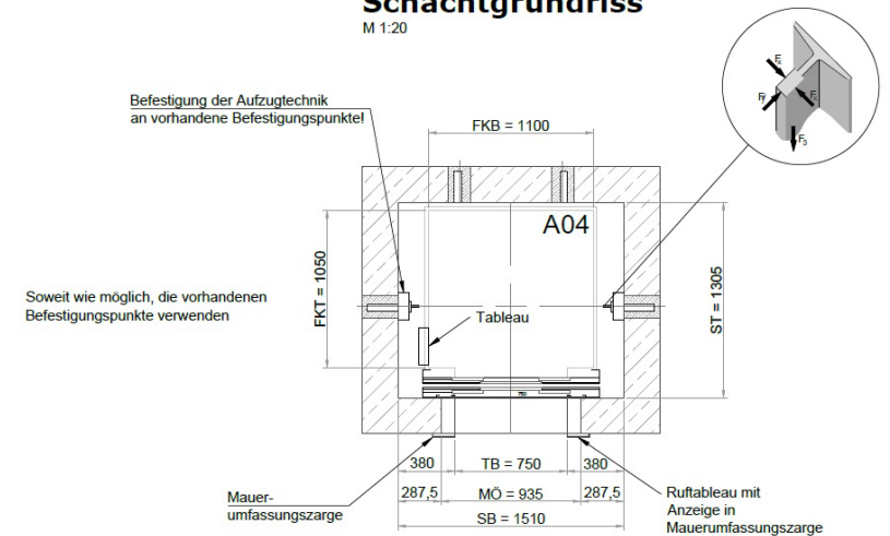
Schachtgrundriss
